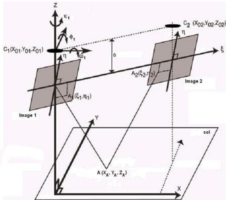
Figure 3. Systèmes de référence et caractéristiques géométriques d'un couple stéréoscopique (d'après Kraus & WALDHÄUSL, 1979 ; JENSEN, 2000 ; CASSON et al., 2005). (X, Y, Z) : système de référence absolu ; C_1 (X_{01}, Y_{01}, Z_{01}) et C_2 (X_{02}, Y_{02}, Z_{02}) : positions 1 et 2 de la caméra dans le repère absolu de référence ; (\eta, \xi) : repère "image" de référence ; A_1 et A_2 : points "images" correspondant au point au sol A ; c : distance focale de l'objectif ; (\omega, \phi, \kappa) : angles de rotation de la caméra.
