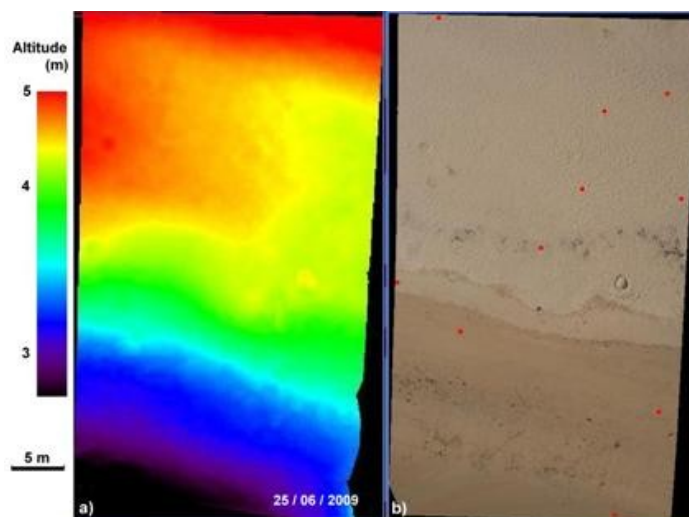
Figure 4. MNT (a) et ortho-image (b) générés à partir d'un couple d'images acquises lors de la mission Porsmilin du 25/06/2009.
