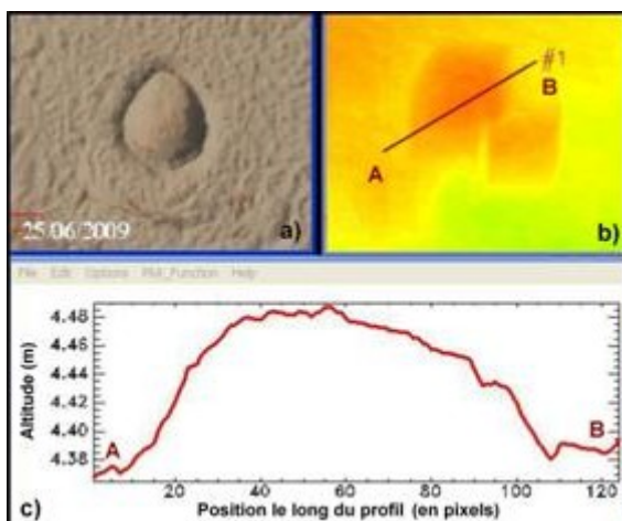
Figure 7. Zoom sur un détail: une plate-forme de sable d'environ 1,5m de diamètre visualisée sur l'ortho-image (a), le MNT (b) et le profil en coupe verticale (c).
