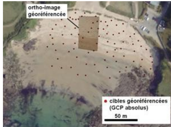
Figure 5. Ortho-image géoréférencée insérée dans un SIG.
