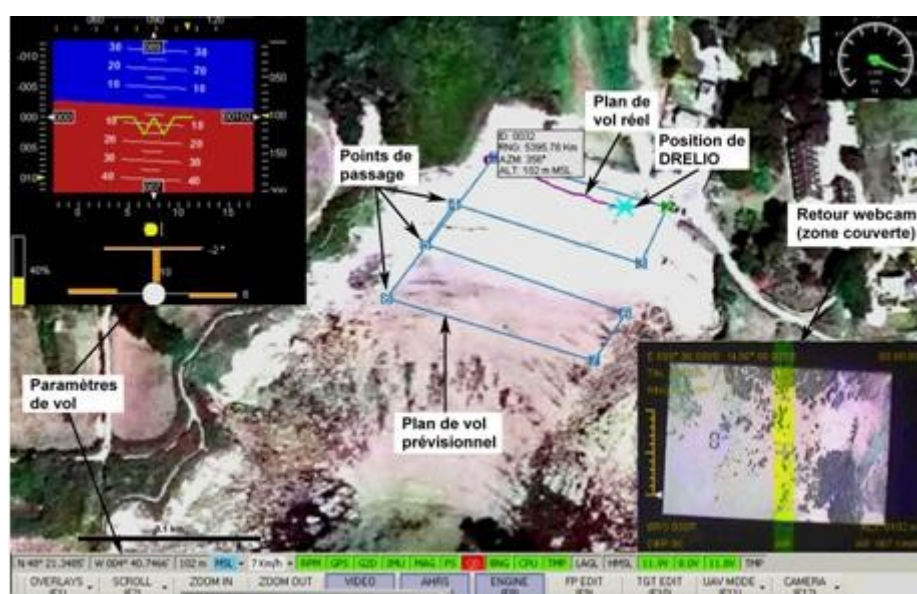
Figure 2. Ecran de contrôle de l'auto-pilote.
