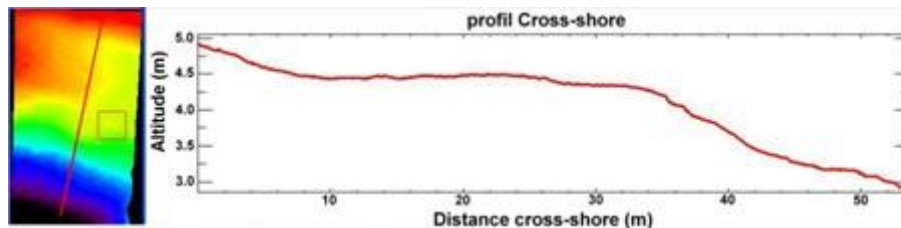
Figure 6. Profil transversal selon Z sur le MNT généré précédemment.
